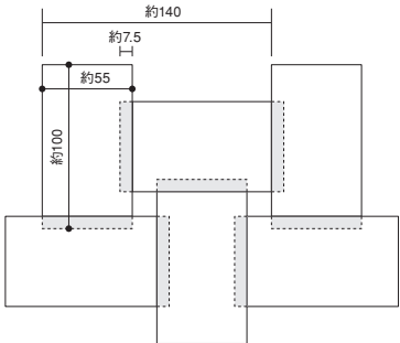
施工図
